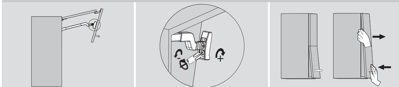
Montagem da porta
