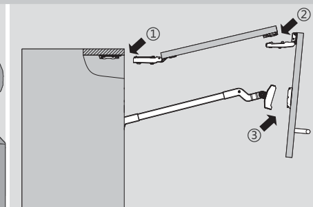
Montagem da porta
