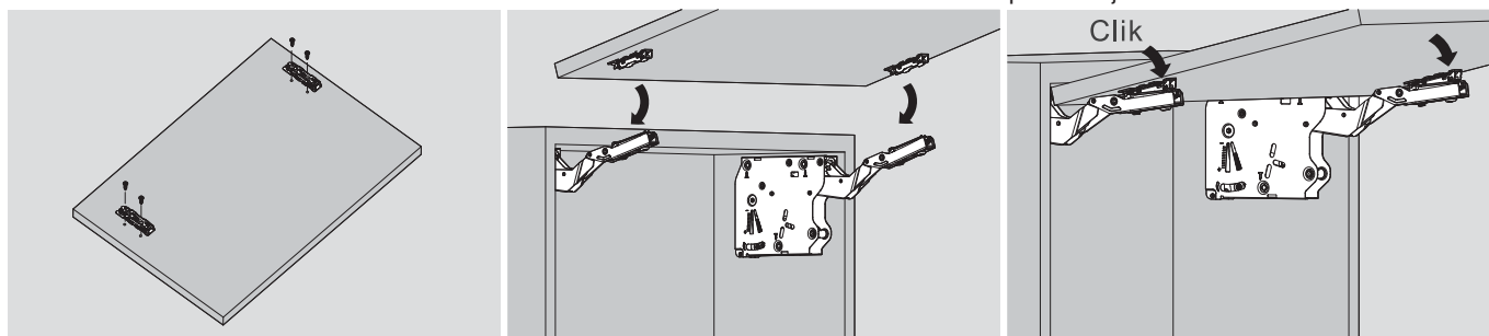
Instalação do fixador do painel
