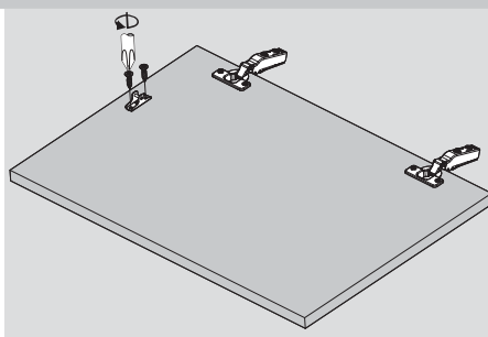
Montagem da porta
