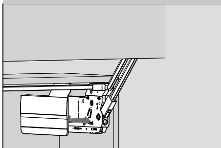
Montagem da tampa de acabamento
