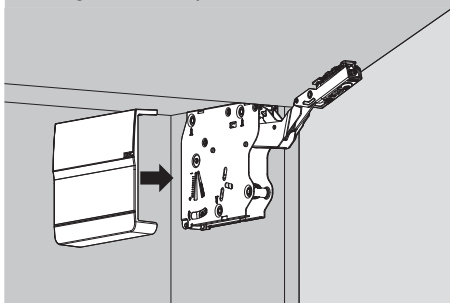
Montagem das tampas
