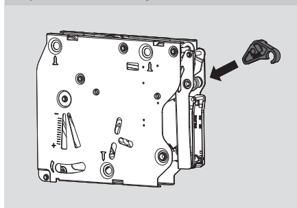
Clipe limitador do ângulo de abertura
