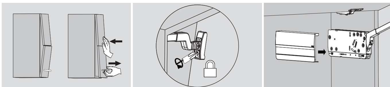
Ajuste do posicionamento das portas
