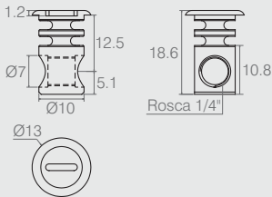
Porca Cilíndrica com Cabeça 09.01.105
